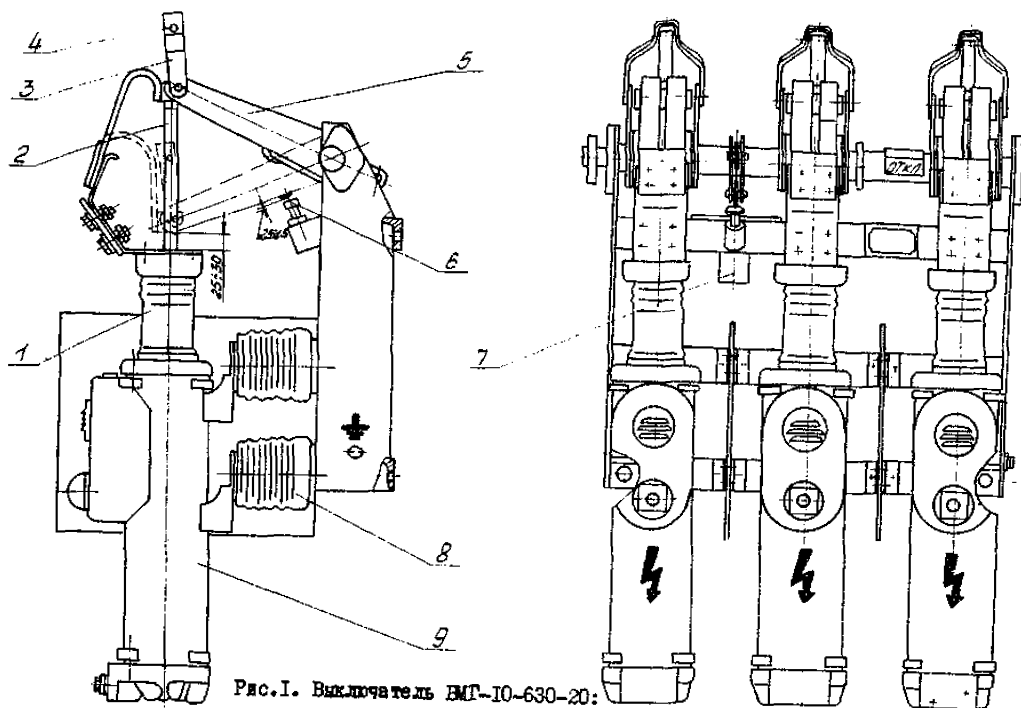
Рис.1. Выключатель ВМП-10-630-20: 1 - проходной изолятор; 2 - контактные стержни; 3 - серьга; 4 - ось; 5 - изоляционный рычаг; 6 - болт - упор; 7 - масляный буфер; 8 - опорный изолятор; 9 - сек.
