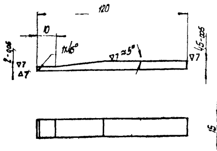
Рис. 11. Шаблон П1 для измерения хода релейной полки в пределах 2,0-4,5 мм
