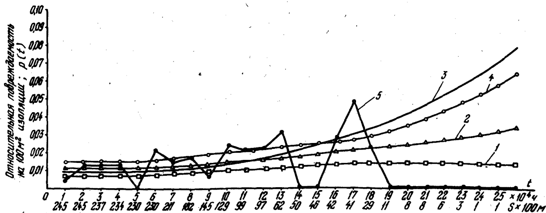
Рис. П2. I. Текущая кривая вероятности аварийного пробоя изоляции некоторой совокупности генераторов с воздушным охлаждением:
