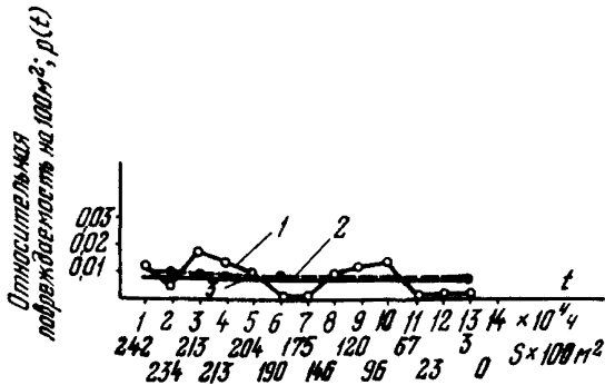
Рис. III.3. Текущая кривая вероятности аварийного пробоя изоляции обмоток статоров ТГВ-200 ( по состоянию на I.01.1979 г.):
