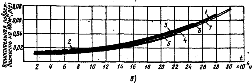
Рис. П1.7. Текущие кривые вероятности аварийного пробоя микалентной изоляции генераторов наблюдаемой совокупности, работающей в воздушной среде:
