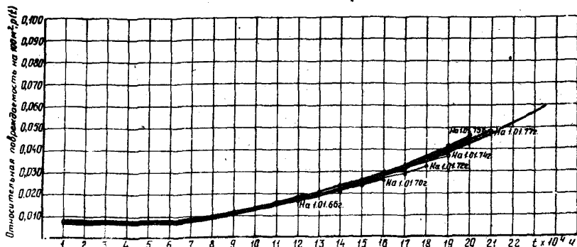
Рис. П.1.6. Текущие кривые вероятностей аварийного пробоя изоляции гидрогенераторов 13,8 кВ за минусом генераторов СВ-1160/180-72, установленных на электростанциях № 16 и 5 и с учетом поправки по электростанции № 3
