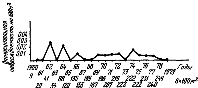
Рис. П.2. Календарный график аварийной повреждаемости изоляции обмоток статоров ТГВ-200
