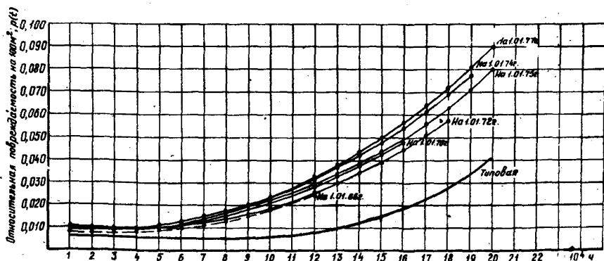
Рис. III.5. Текущие кривые вероятностей аварийного пробоя изоляции всей совокупности гидрогенераторов 13,8 кВ
