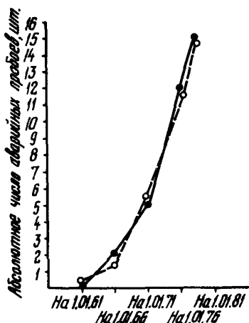
Рис. III.4. Динамика соотношений ожидаемого и фактического числа аварийных пробоев ТГВ-200 ( за период 1960-1978гг)
