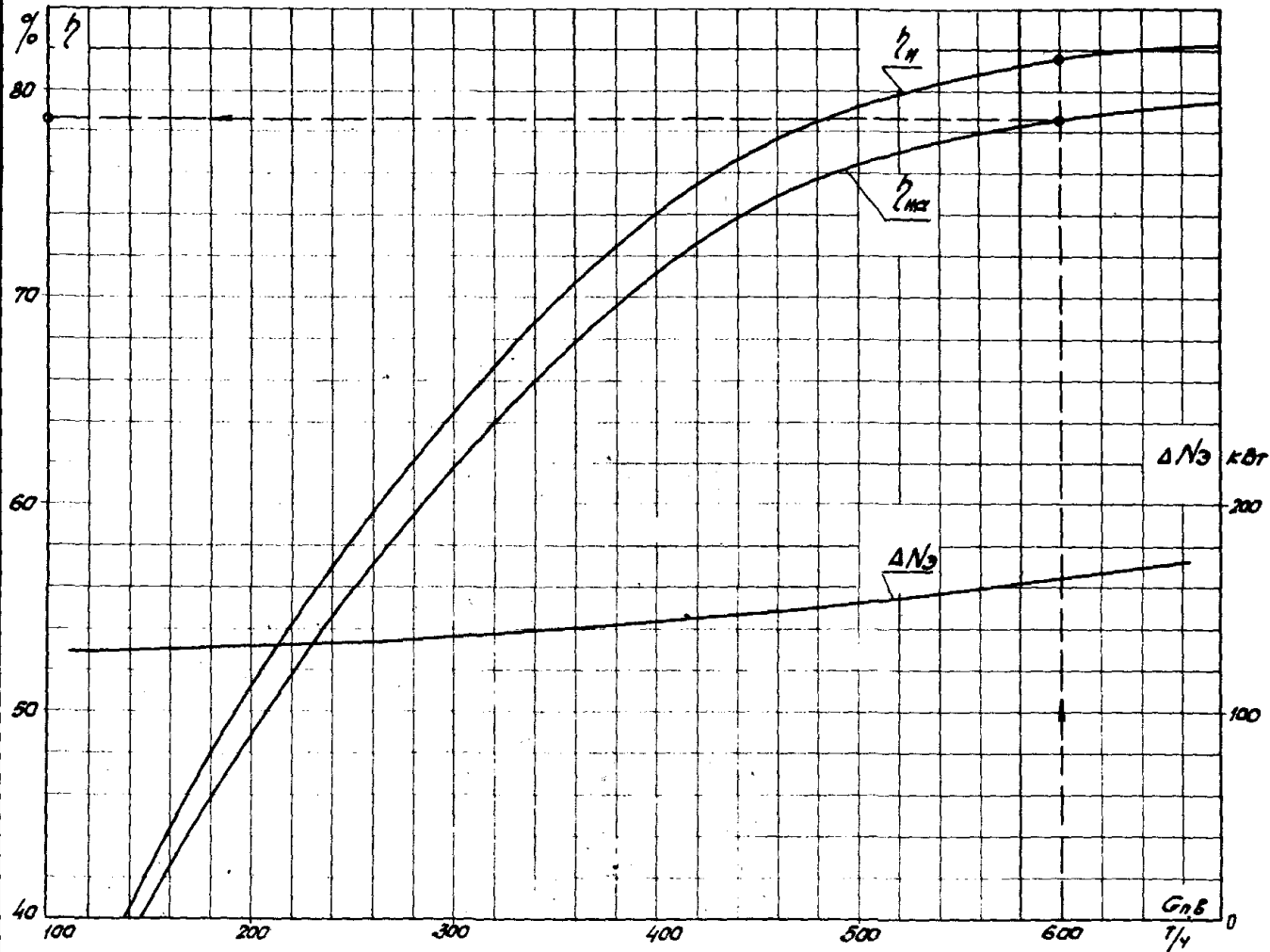
Т-3 Типовая энергетическая характеристика питающего электронасоса. КПД насоса, насосного агрегата и потери в электродвигателе.
