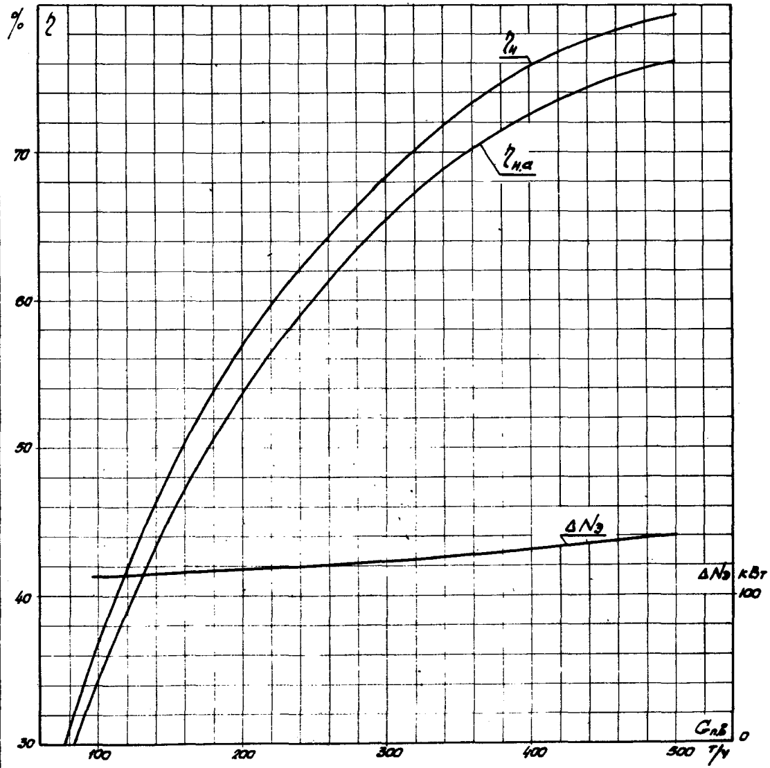
Т-3 Типовая энергетическая характеристика питающего электронасоса КПД насоса, насосного агрегата и потери в электро-двигателе Тип ПЗ-500-180-4
