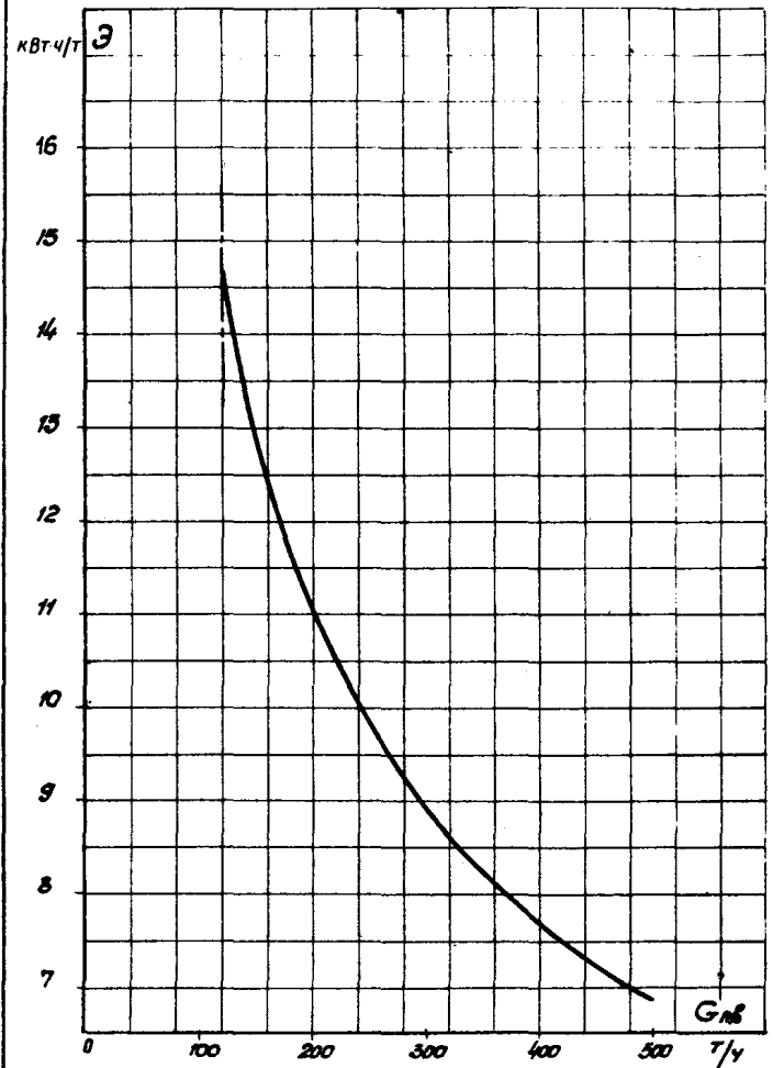
Т-2 Типовая энергетическая характеристика питающего электронасоса. Удельный расход электроэнергии на тонну перекачиваемой воды. Тип ПЗ-500-180-4
