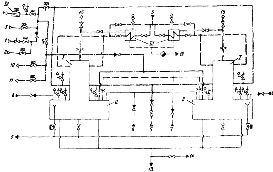
Рис.29. Типовая схема деаэрационной установки энергоблоков I50-200 МВт с колонкой типа ДП-320 (ДП-400, ДП-500):
