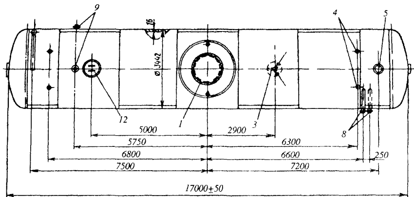
Рис.24. Деаэрационный бак БДП-120-1 объемом 120 \text{ м}^3 для одной колонки ДП-500. (Обозначения см. на рис.22)
