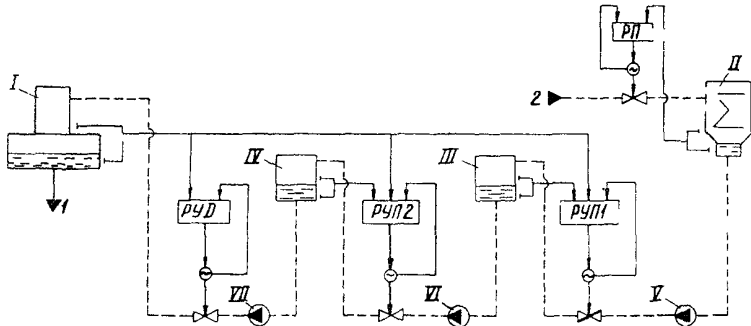
Рис.43. Схема регулирования уровней для энергоблоков мощностью 500 и 800 МВт с продольными конденсаторами:
