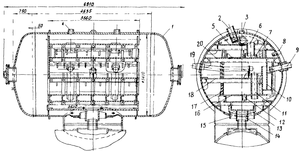
Рис.13. Деаэрационная колонка ДП-1300. (Обозначения см.на рис.12)
