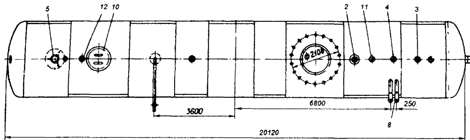
Рис.26. Деаэрационный бак ВДП-150-1 объемом 150 м 3 для колонки ДП-2000:
