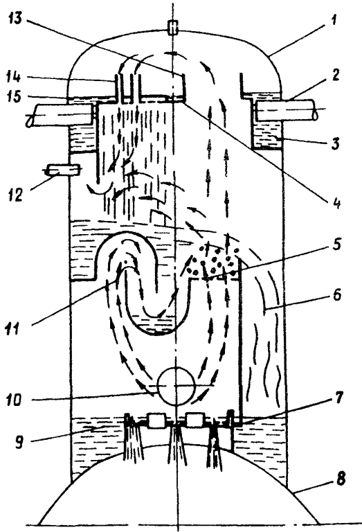
Рис.10. Принципиальная схема деаэрационной колонки ДП-1000:
