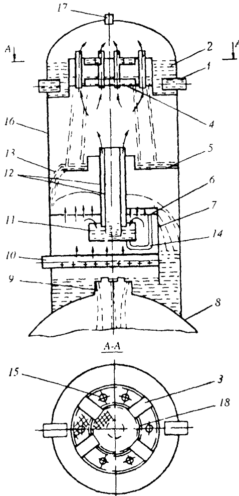
Рис.7. Принципиальная схема колонки ДП-225 (الم-500):
