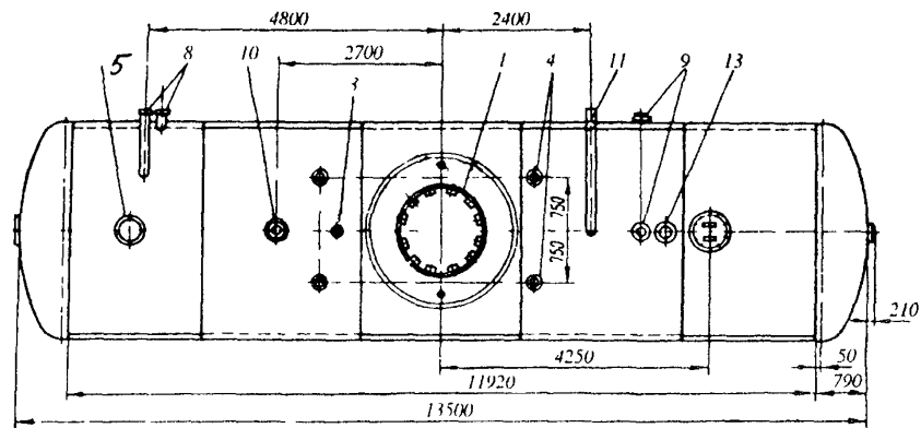
Рис.23. Деаэрационный бак БДП-100-І объемом 100 м 3 для одной колонки ДП-500. (Обозначения см. на рис.22)
