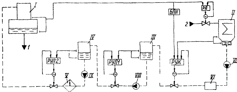
Рис.39. Схема регулирования уровней с дополнительным сигналом по уровню в деаэраторе для блоков КЭС со смешивающими ПНД 1 и 2: I - деаэратор; II - конденсатор; III-IV - подогреватели низкого давления № 1 и 2; У - подогреватели низкого давления № 3 и 4; УI - ВСУ УП-IХ - конденсатные насосы № 1, 2 и 3; I - п.в. на всас ПТН; 2 - конденсат из ВЗК
