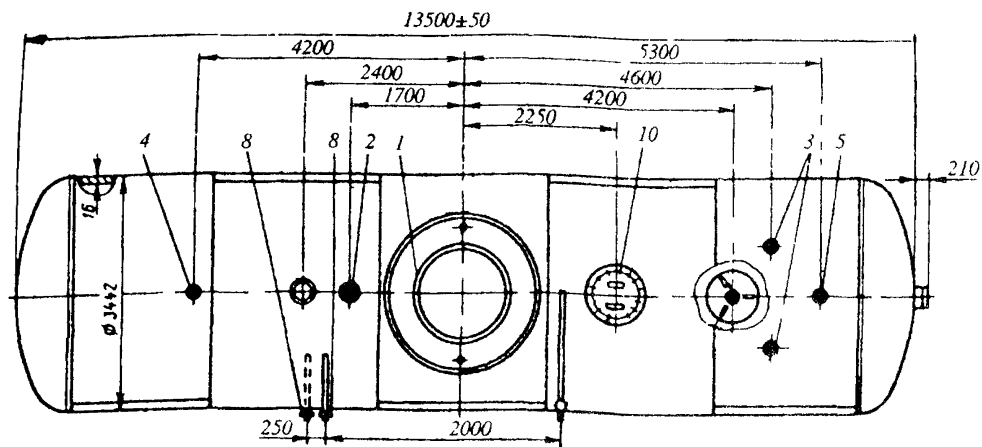
Рис.25. Деаэрационный бак БДП-100-1 объемом 100 м 3 для колонки ДП-1000:
