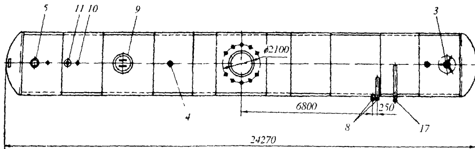
Рис.27. Деаэрационный бак БДП-185-1 объемом 185 м 3 для колонки ДП-2000:
