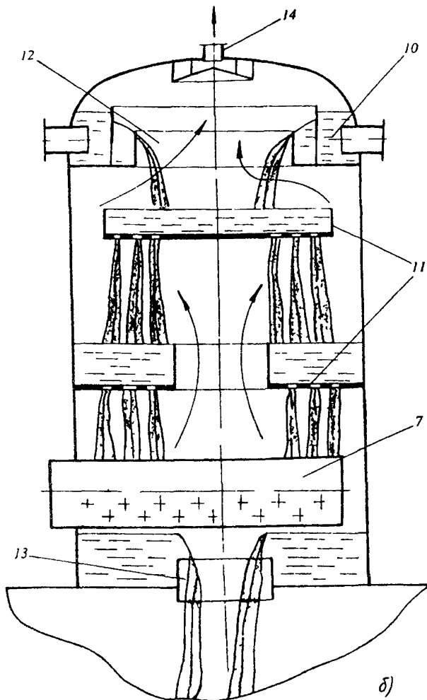
Рис. 3. Деаэрационная колонка струйного типа ДП-800:
