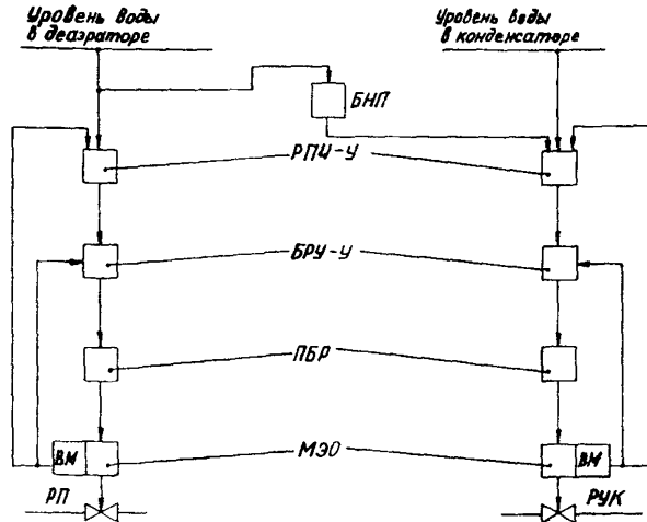
Рис. 41. Структурная схема системы регулирования уровня в деаэраторе и конденсаторе на аппаратуре АКЭСР-П для блока КЭС с поверхностными ПИД:
