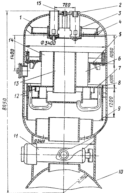
Рис.19. Конструкция деаэрационной колонки ДП-2800. (Обозначения см.на рис.18)
