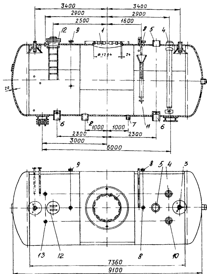
Рис. 22. Деаэрационный бак БДП-65-I объемом 65 м 3 для колонок ДП-225 и ДП-500:
