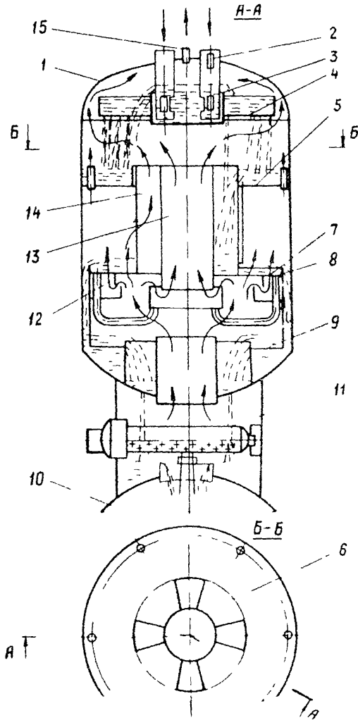
Рис. 18. Принципиальная схема деаэрационной колонки ДП-2800:
