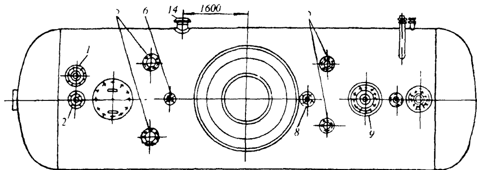
Рис.20. Бак-аккумулятор объемом 65 \text{ м}^3 для колонки ДП-500:
