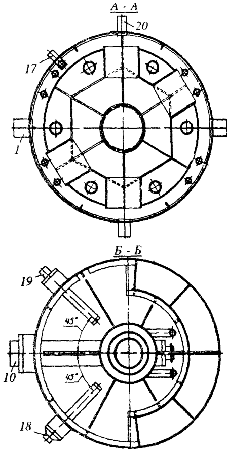
Рис.9. Деаэрационная колонка ДП-500: 18 - ввод пара от расширителя; 19 - ввод пара от штоков клапана; 20 - ввод воды от уплотнений (Остальные обозначения см.на рис.7)
