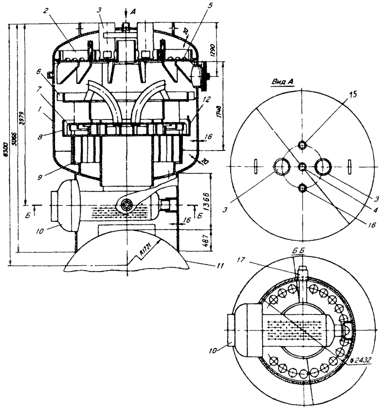
Рис.17. Деаэрационная колонка ДП-2000: 15 - ввод воды от уплотнений ПТН; 16 - ввод воды от уплотнений ПСН; 17 - ввод пара от штоков клапанов (Остальные обозначения см.на рис.14)
