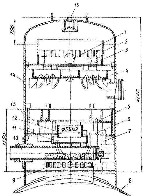
Рис.6. Деаэрационная колонка ДШ-1000 струйно-барботажного типа. (Обозначения см.на рис.4)
