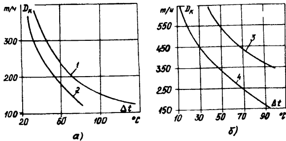
Рис.2. Характеристики предельных режимов деаэраторов:
