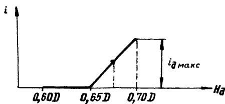
Рис. 42. Характеристика блока БНП в схеме регулирования уровня с дополнительным сигналом по уровню в деаэраторе для блоков КЭС со смешивающим ПНД-2
