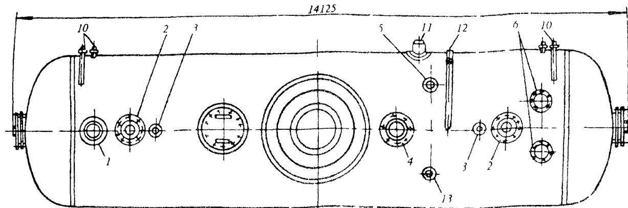
Рис.21. Бак-аккумулятор объемом 100 м 3 для колонки ДГ-800:
