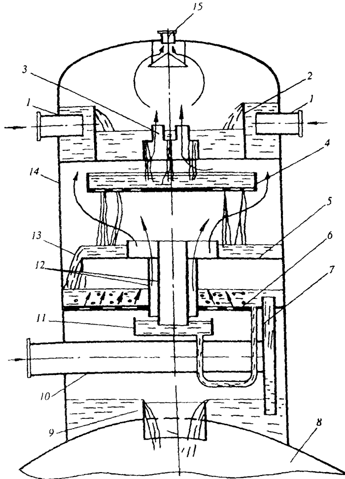
Рис.4. Принципиальная схема деаэрационной колонки ДП-500М:
