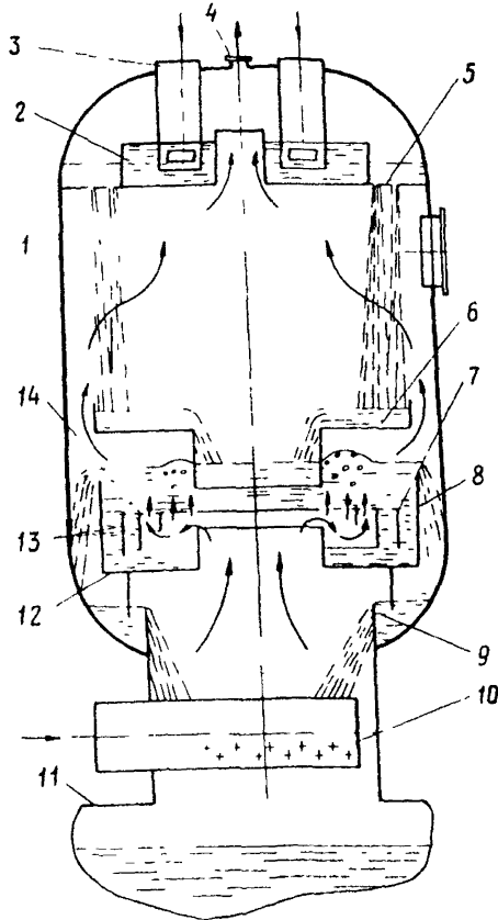
Рис.14. Принципиальная схема деаэрационной колонки ДП-2000-I:
