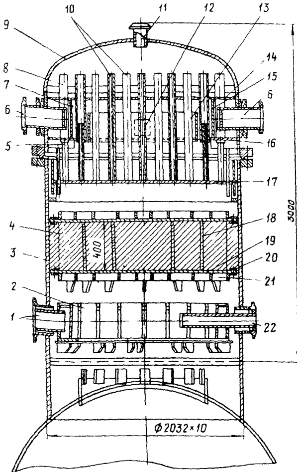
Рис. 1. Деаэрационная колонка ДП-320:
