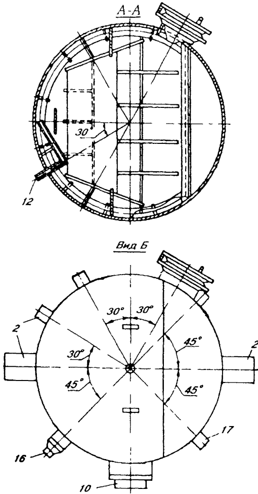
Рис. II. Деаэрационная колонка ДП-1000: 16 - ввод пара от штоков и клапанов; 17 - рециркуляция бустерных насосов; 18 - конденсат от уплотнений питательных насосов; 19 - воздушник
