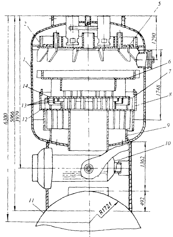
Рис. 15. Конструкция деаэрационной колонки ДП-2000-I. (Обозначения см. на рис. 14)
