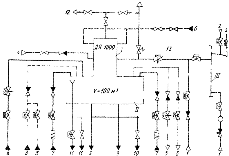
Рис.32. Типовая схема деаэрационной установки с колонкой ДП-1000 теплофикационного дубль-блока с турбиной Т-185/220-130 и барабанными котлами:
