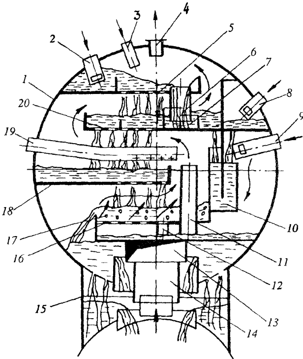
Рис. 12. Принципиальная схема деаэрационной колонки ЛД-1300:
