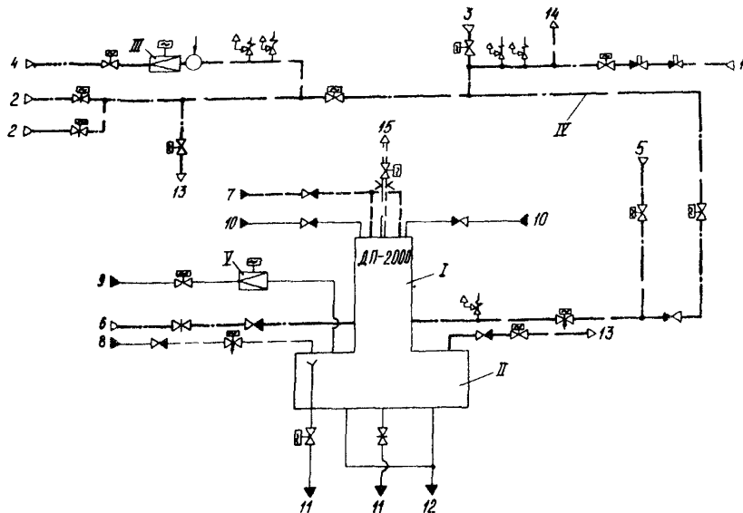
Рис.35. Типовая схема деаэрационной установки моноблока 500 МВт с колонкой типа ДП-2000: I - деаэрационная колонка; II - бак-аккумулятор; Ш - РОУ 40/13; IУ - коллектор собственных нужд (КСН); У - дроссельный клапан;
