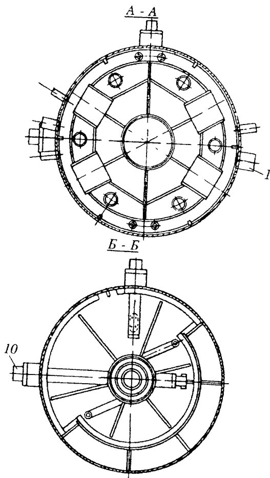
Рис.8. Деаэрационная колонка ДП-225. (Обозначения см.на рис.7)
