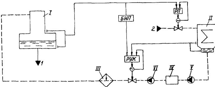
Рис.40. Схема регулирования уровней с дополнительным сигналом по уровню в деаэраторе для блоков КЭС с поверхностными ПНД: I - деаэратор; II - конденсатор; III - подогреватели низкого давления; УI - ВСУ; У-II - конденсатные насосы № 1 и 2; I - п.в. на всас ПТН; 2 - конденсат из ВЗК
