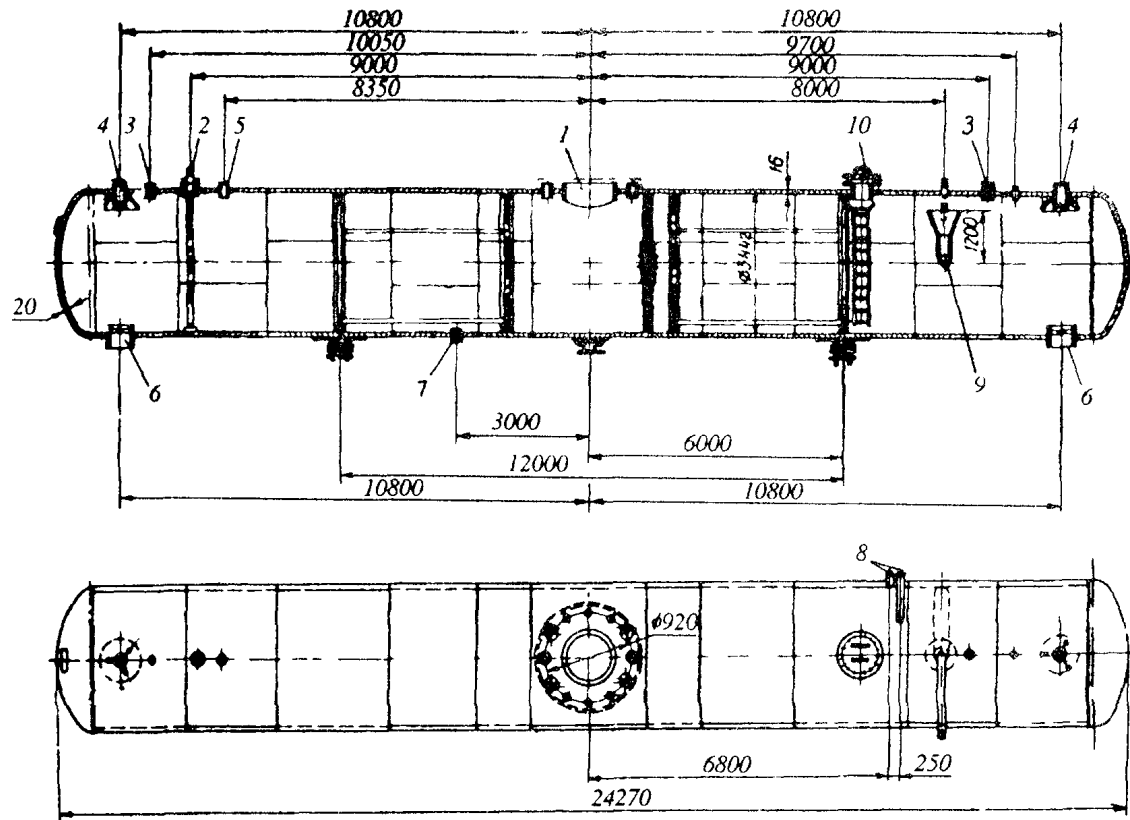
Рис.28. Деаэрационный бак БДП-185-1 объемом 185 м 3 для колонки ДП-2800 (Обозначения см. на рис.25)
