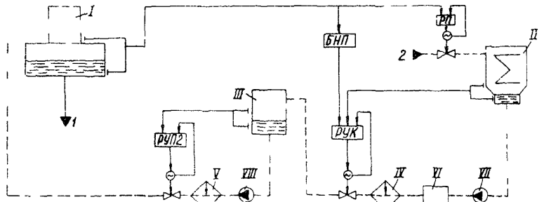
Рис.38. Схема регулирования уровней с дополнительным сигналом по уровню в деаэраторе для блоков КЭС со смешивающим ПНД-2: I - деаэратор; II - конденсатор; III - подогреватель низкого давления № 2; IV и V - подогреватели низкого давления № 1 и № 3 и 4; У1 - БОУ; УП-УШ - конденсатные насосы № 1 и 2; I - п.в. на всас ПТН; 2 - конденсат из БЗК
