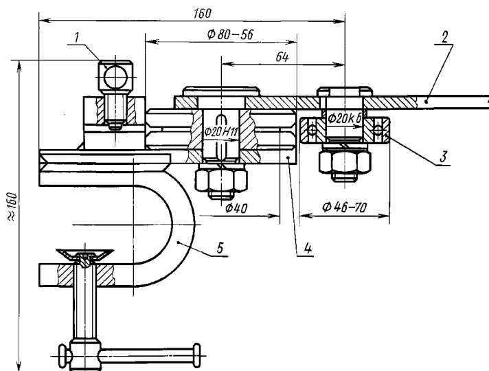
1 — винт; 2 — рукоятка; 3 — огибающий ролик; 4 — гибочный ролик; 5 — скоба
