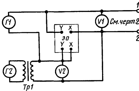
Схема включения аппаратуры для испытания приборов на влияние формы кривой напряжения или тока
