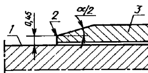
1 — поверхность стебля; 2 — измерительная кромка; 3 — барабан
