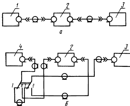
Схема проверки ослабления взаимной модуляции
