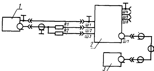
1 — генератор синусоидальных сигналов; 2 — эквивалент сети; 3 — измеритель радиопомех; R_1 = R_2 = 150 \pm 1,5 Ом; Ш1, Ш4 — разъемы «ЗЕМЛЯ»; Ш2, Ш3 — разъемы «ИСТОЧНИК РАДИОПОМЕХ»; Ш5, Ш6 — разъемы «СЕТЬ ЭЛЕКТРОПИТАНИЯ»; Ш7 — разъем «ИЗМЕРИТЕЛЬ РАДИОПОМЕХ»
