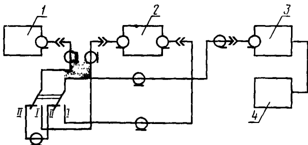
1 — генератор синусоидальных сигналов; 2 — режекторный фильтр; 3 — аттенюатор; 4 — вольтметр переменного тока
