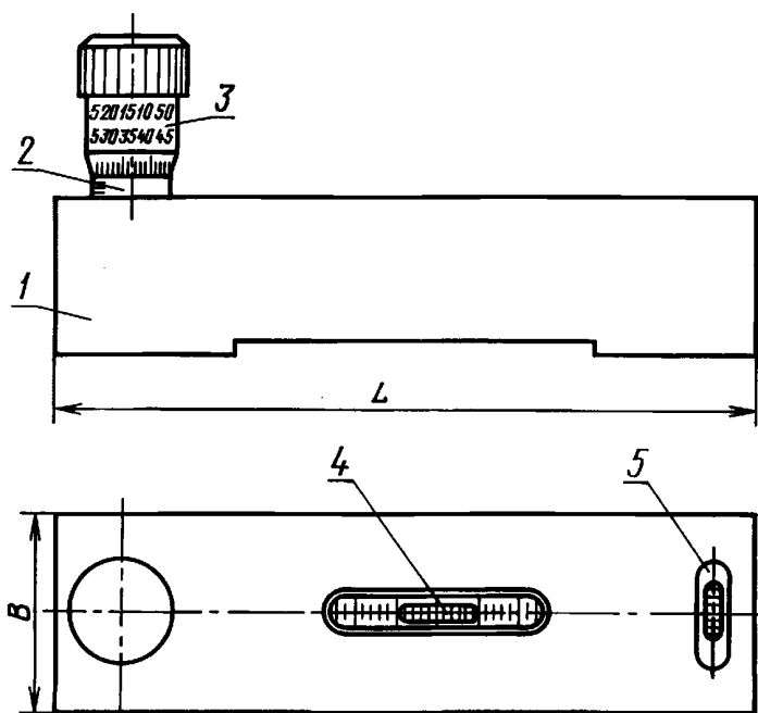
1 — основание; 2 — стебель; 3 — барабан; 4 — продольная ампула; 5 — поперечная ампула
