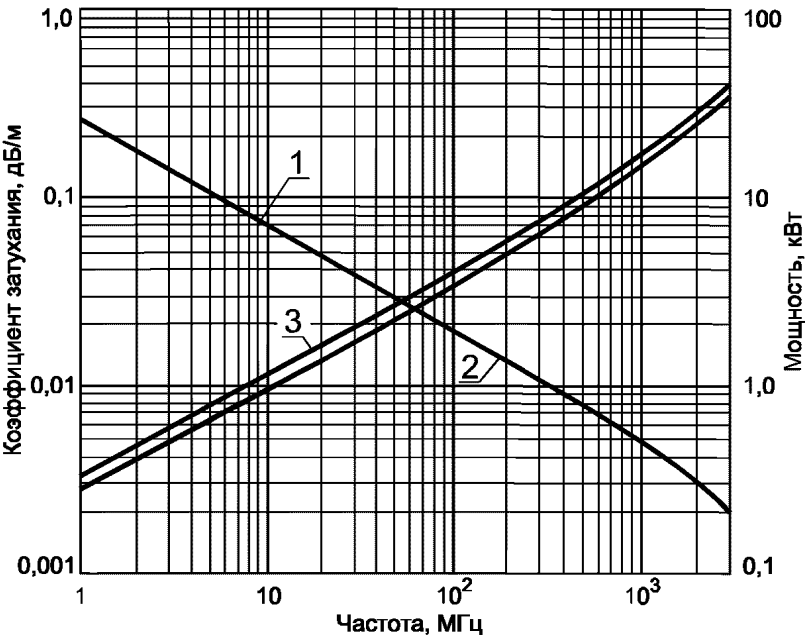
Частотные зависимости
