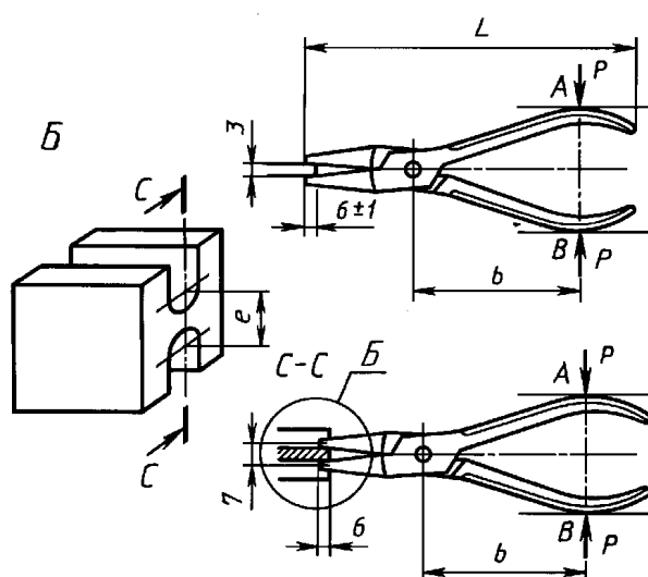
Рисунок 13 — Изолирующие плоскогубцы и круглогубцы. Испытание на кручение
