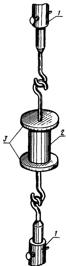
1 — зажим; 2 — образец; 3 — пластины
