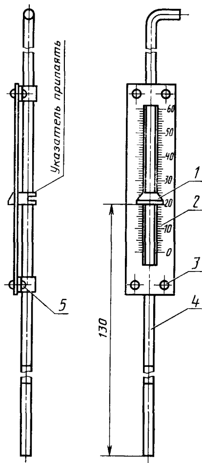
Пластометр
