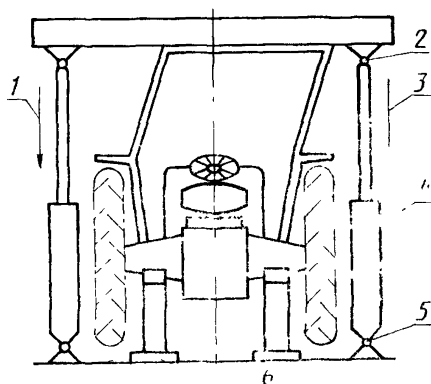
Пример приспособления для приложения вертикальной статической нагрузки
