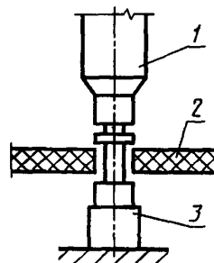
1 — машина; 2 — пол; 3 — нагрузочное устройство
