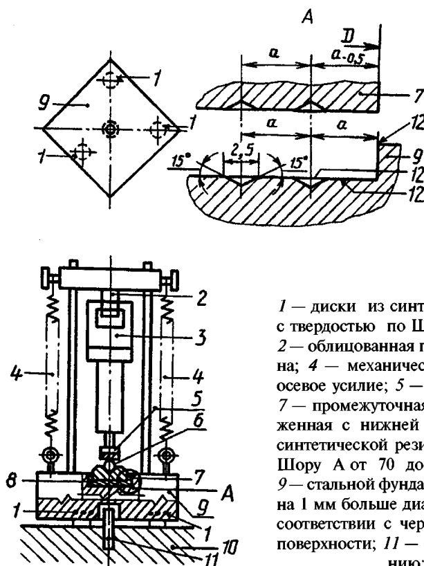
Испытательный прибор
