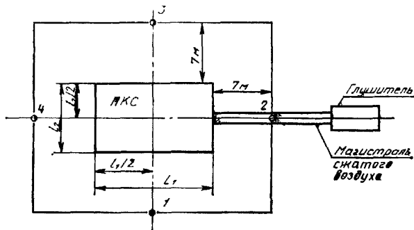
1—4 — точки измерения шума, l_1 и l_2 — длина и ширина гибкого источника шума параллелепипеда
