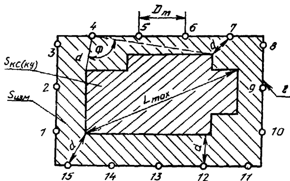
1—16 — точки измерения; \Phi — угол обзора; D_m — расстояние между точками измерения; d — измерительное расстояние; L_{\text{max}} — наибольший размер по площади КС (КУ); S_{\text{КС(КУ)}} — площадь КС (КУ); S_{\text{изм}} — измерительная площадь; l — длина измерительного контура
