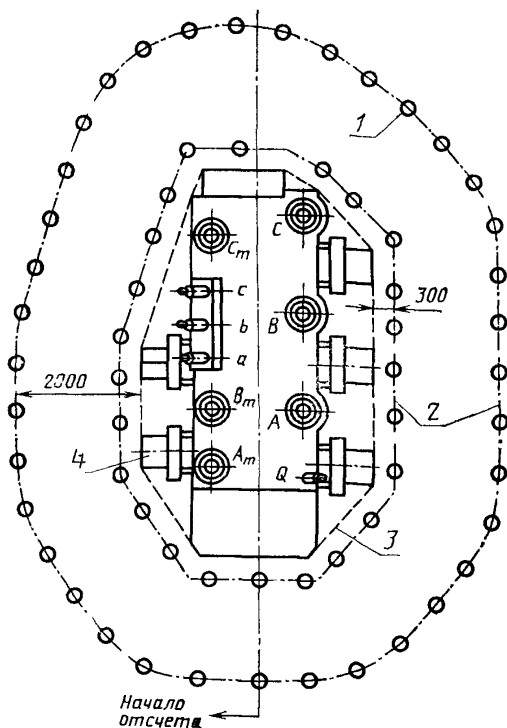
1 — микрофон; 2 — измерительная линия; 3 — излучающая поверхность; 4 — охладитель
