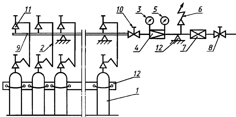
г) Рампа с баллонами, соединенными в группу
