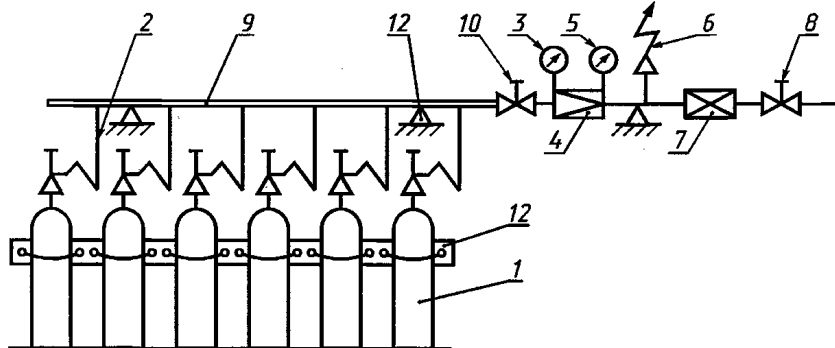
в) Рампа с более 6 баллонами
