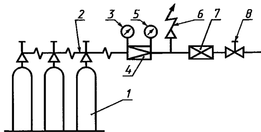
б) Рампа с 6 и менее баллонами
