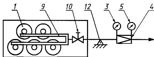
г) Рампа с баллонами, соединенными в группу
