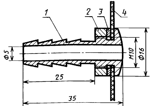
1 — штуцер; 2 — гайка; 3 — шайба; 4 — лицевая часть СИЗОД
