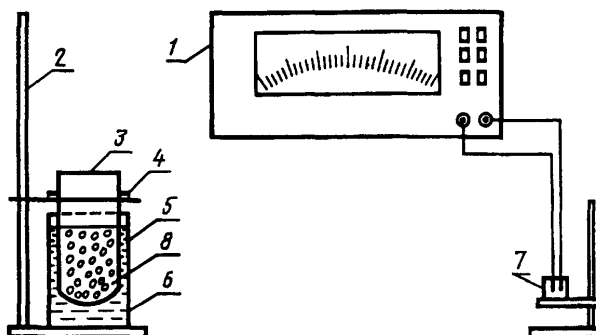
1 — рН-метр-милливольметр; 2 — штатив с кольцом; 3 — изделие; 4 — стержень; 5 — емкость вместимостью 3 л; 6 — агрессивная жидкость; 7 — стакан для отбора проб; 8 — жидкость в изделии
