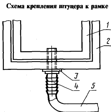
1 — рамка; 2 — изоляция термостабильной плиты; 3 — прокладка; 4 — штуцер; 5 — резиновая трубка
