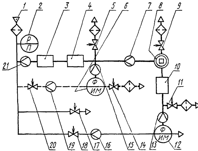
Принципиальная схема установки для контроля фильтрующих коробок по коэффициенту проскока масляного тумана
