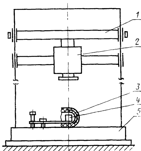
1—каретка; 2—боек; 3—носик; 4—пластилиновый столбик; 5—основание
