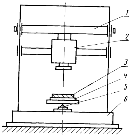
1—каретка; 2—боек; 3—защитный элемент; 4—плата; 5—датчик; 6—основание
