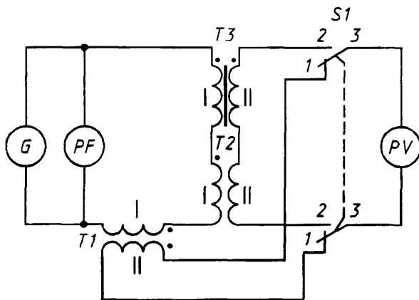
Рисунок 1 — Схема для измерений в динамическом режиме перемангничивания
