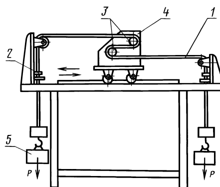
1 — испытуемый образец; 2 — ограничивающие зажимы; 3 — сменные ролики; 4 — каретка; 5 — груз
