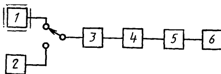
1 — передатчик; 2 — высокочастотный генератор сигналов; 3 — испытательная нагрузка передатчика; 4 — аттенюатор; 5 — режекторный фильтр; 6 — измерительный приемник (табл. 6, п. 11)
