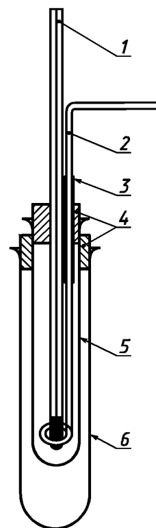
1 — термометр; 2 — гибкая проволочная мешалка; 3 — стеклянная трубка; 4 — пробки; 5 — пробирка; 6 — рубашка
