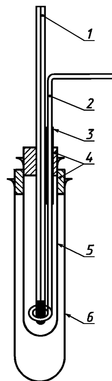
1 — термометр; 2 — гибкая проволоочная мешалка; 3 — стеклянная трубка; 4 — пробка; 5 — пробирка; 6 — рубашка
