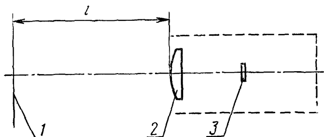
1 — экран испытываемого аппарата; 2 — объектив или линза, 3 — элемент, корригированный на спектральную чувствительность глаза человека ( v(\lambda) )
