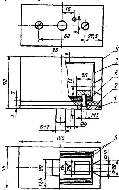
1—стальное основание камеры с фиксаторами; 2—асбестоцементная плита; 3—стальная коробка; 4—теплоизоляция; 5—миканит; 6—электронагреватель
