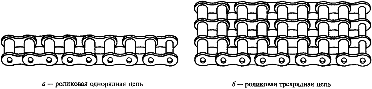
Рисунок А.1 — Типы роликовых цепей в сборе
