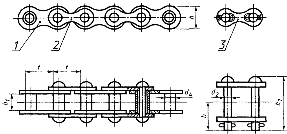
1 — внутреннее звено; 2 — наружное звено; 3 — соединительное звено Рисунок 5 — Цепь типа ПВ
