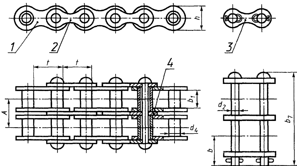
1 — внутреннее звено; 2 — наружное звено; 3 — соединительное звено; 4 — промежуточная пластина Рисунок 6 — Цепь типа 2ПВ
