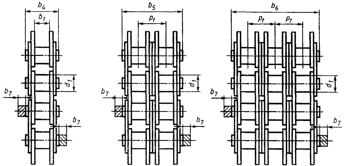
г — однорядная цепь д — двухрядная цепь е — трехрядная цепь
