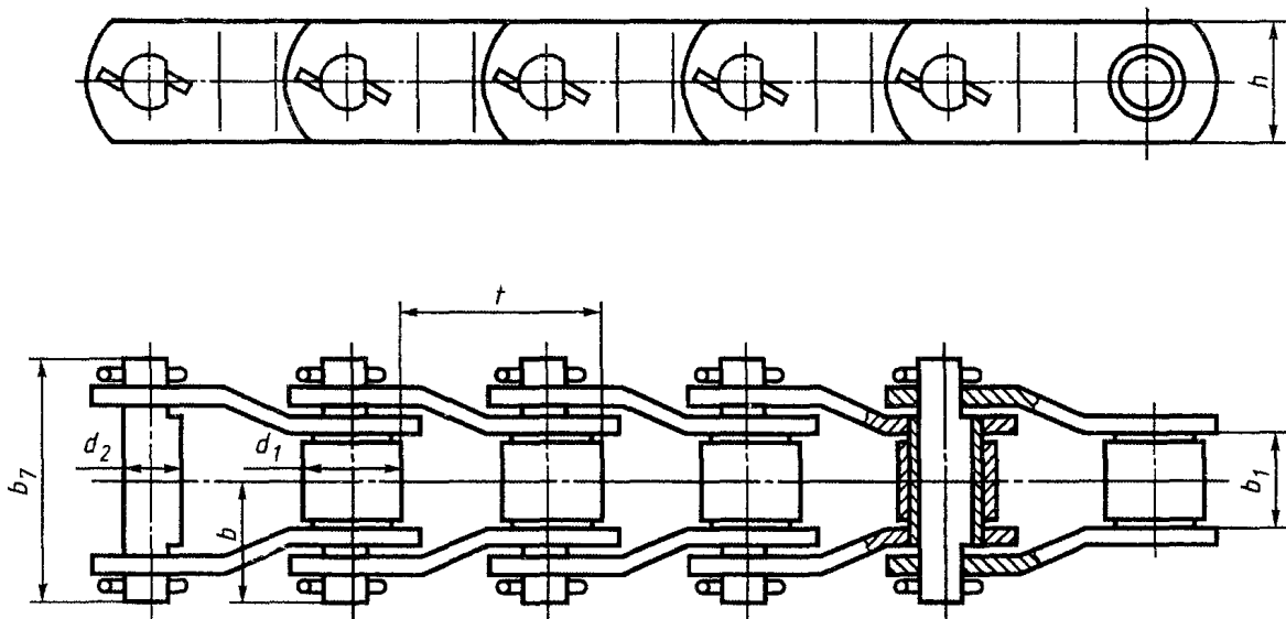
Рисунок 7 — Цепь типа ПРИ
