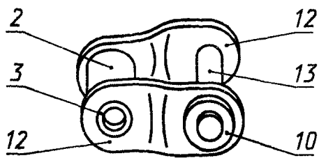
е — переходное звено однорядное
