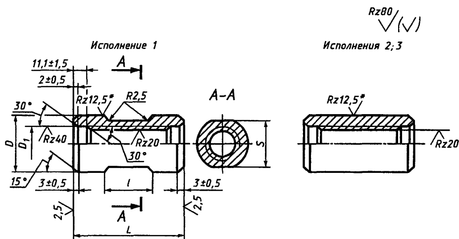
Рисунок 3 — Соединительная муфта
