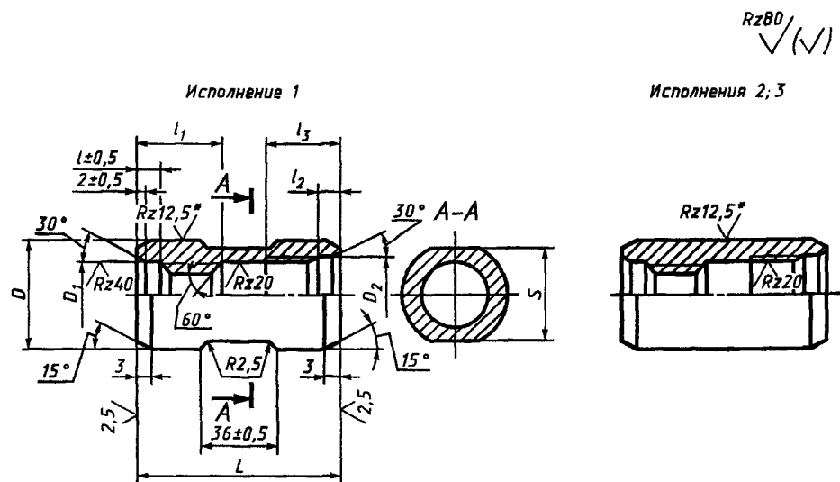
Рисунок 4 — Переводная муфта
