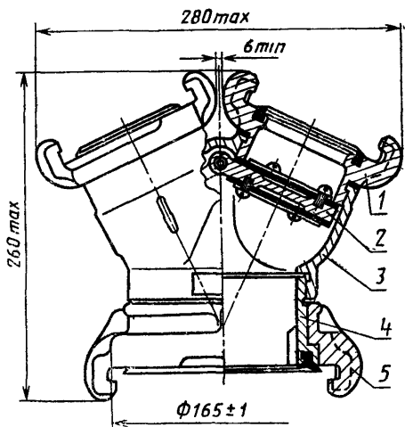
1; 5—соединительные головки; 2—клапан; 3—корпус; 4— выходной патрубок
