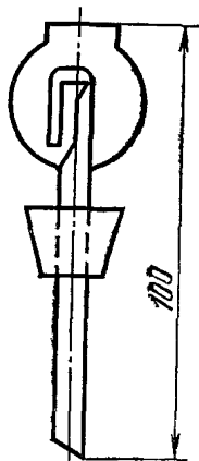
Затвор Геккеля
