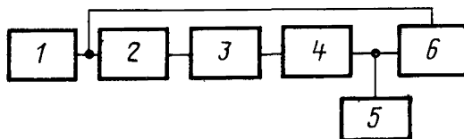
1—генератор сигналов НЧ; 2—датчик испытательных сигналов; 3—генератор сигналов ВЧ; 4—приемник, 5—эквивалент нагрузки; 6—измеритель краевых искажений
