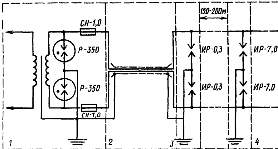
1 — станция; 2 — кабельный ввод; 3 — выводная опора; 4 — фидерная линия
