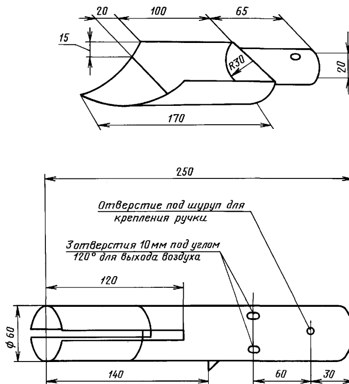
Щуп для отбора точечных проб
