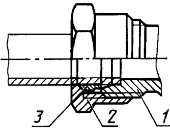
1 — присоединительный конец корпусной детали исполнения 1 по ГОСТ 22525, 2 — накидная гайка по ГОСТ 23353, 3 — врезающееся кольцо по ГОСТ 23354
