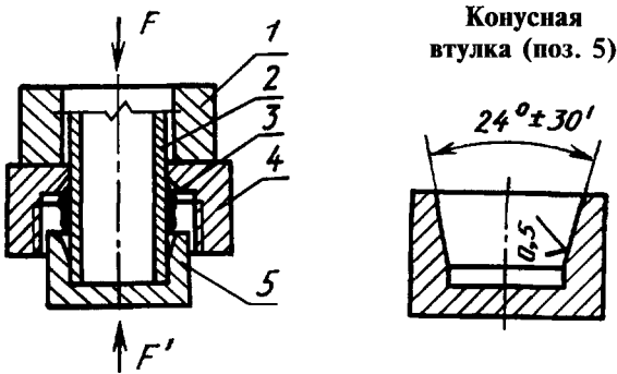
1 — пуансон, 2 — труба, 3 — врезающееся кольцо, 4 — накидная гайка, 5 — конусная втулка
