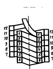
Двухслойная цилиндрическая обмотка трансформатора (к термину 7.2.5)
