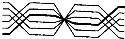
Виды транспозиции (к терминам 7.2.16 и 7.2.17)
