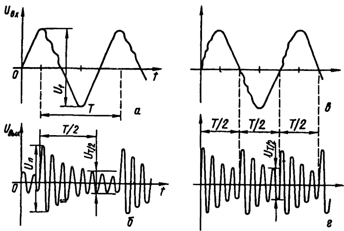
U_{вх} (а, в) – сигнал на входе фильтра ФВЧ; U_{вых} (б, г) – сигнал искажений (призвук) на выходе фильтра ФВЧ; T – период возбуждающего сигнала; U_{п} – двойное амплитудное значение (размах) сигнала призвука на выходе ФВЧ; U_{T/2} – размах сигнала призвука через T/2 после его начала; U_f – размах сигнала на входе ФВЧ на частоте возбуждения громкоговорителя
