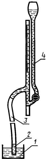
Схема установки для определения количества раствора, протекающего через ключ
