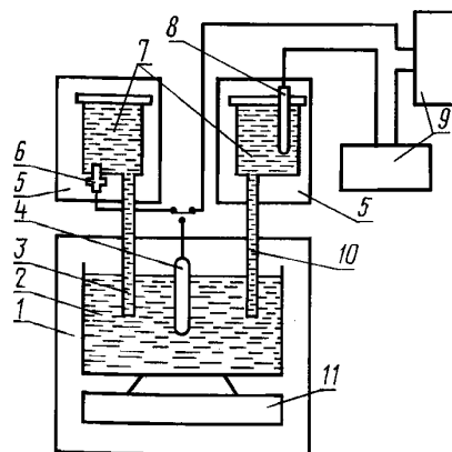
Схема установки для определения потенциала электродов
