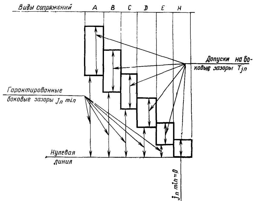
Виды сопряжений и гарантированные боковые зазоры
