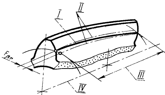
I — действительная делительная линия зуба; II — номинальные делительные линии зуба; III — ширина зубчатого венца; IV — рабочая ось зубчатого колеса.
