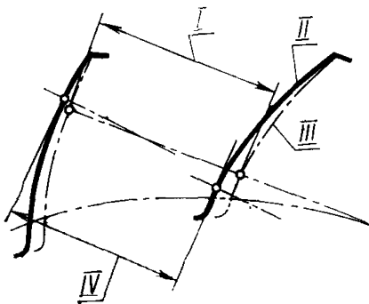
I — номинальный шаг зацепления; II — действительный профиль зуба; III — номинальный профиль зуба; IV — действительный шаг зацепления.
