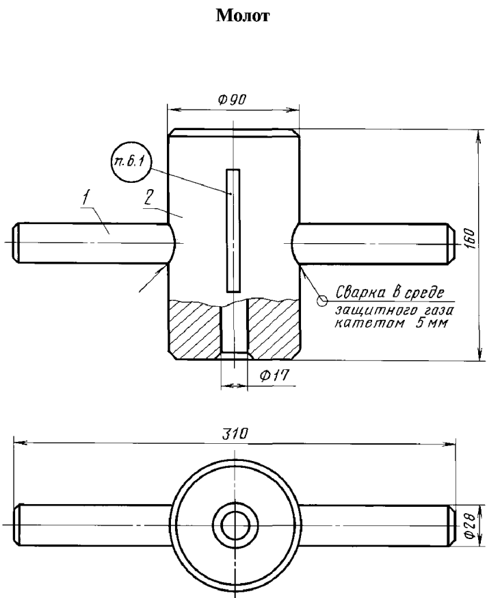
1 — рукоятка; 2 — молот
