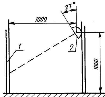
1 — радиометр; 2 — электрокамин
