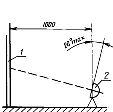
1 — радиометр; 2 — электрокамин
