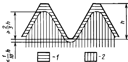
1 — полностью или частично обезуглероженная зона; 2 — необезуглероженная зона
