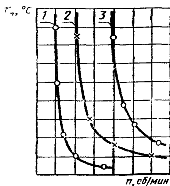
1, 2, 3—при различных \varphi_{\text{окр}} = \text{const} Черт. 23
