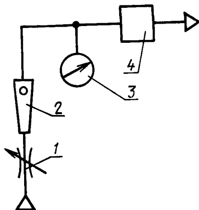
1—дрессель; 2—ротаметр; 3—манометр; 4—аппарат (предохранительный клапан)
