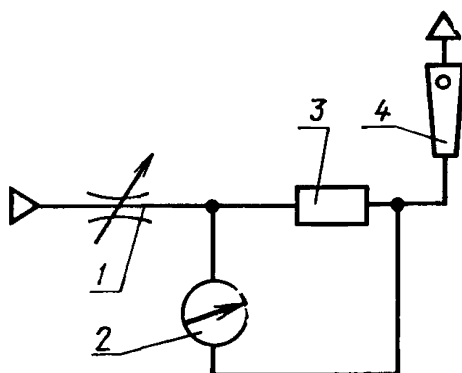
1—дрессель; 2—манометр; 3—аппарат; 4—ротаметр.
