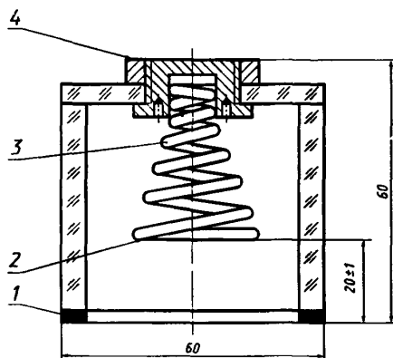
1 — прокладки; 2 — пластина; 3 — пружина; 4 — контакт
